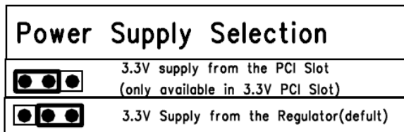
Obrázek 2e - Přepínač E - Nastavení technologie napájení
