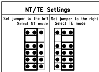
Obrázek 2a - Přepínač A - Nastavení režimu NT nebo TE
