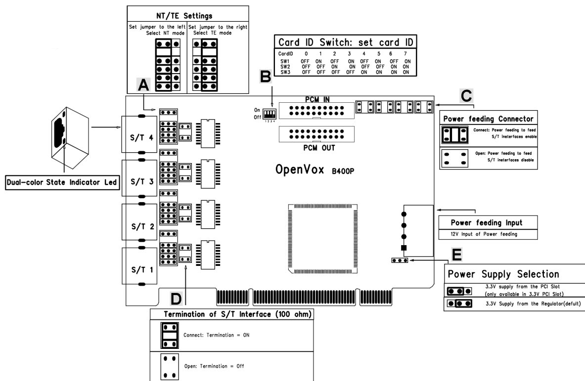
Obrázek 2 - porty a HW přepínače karty
