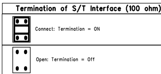
Obrázek 2d - Přepínač D - Propojení zakončovacích odporů na sběrnici
