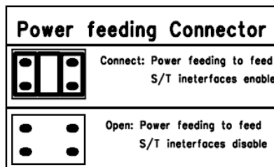
Obrázek 2c - Přepínač C - Propojení napájení na sběrnici
